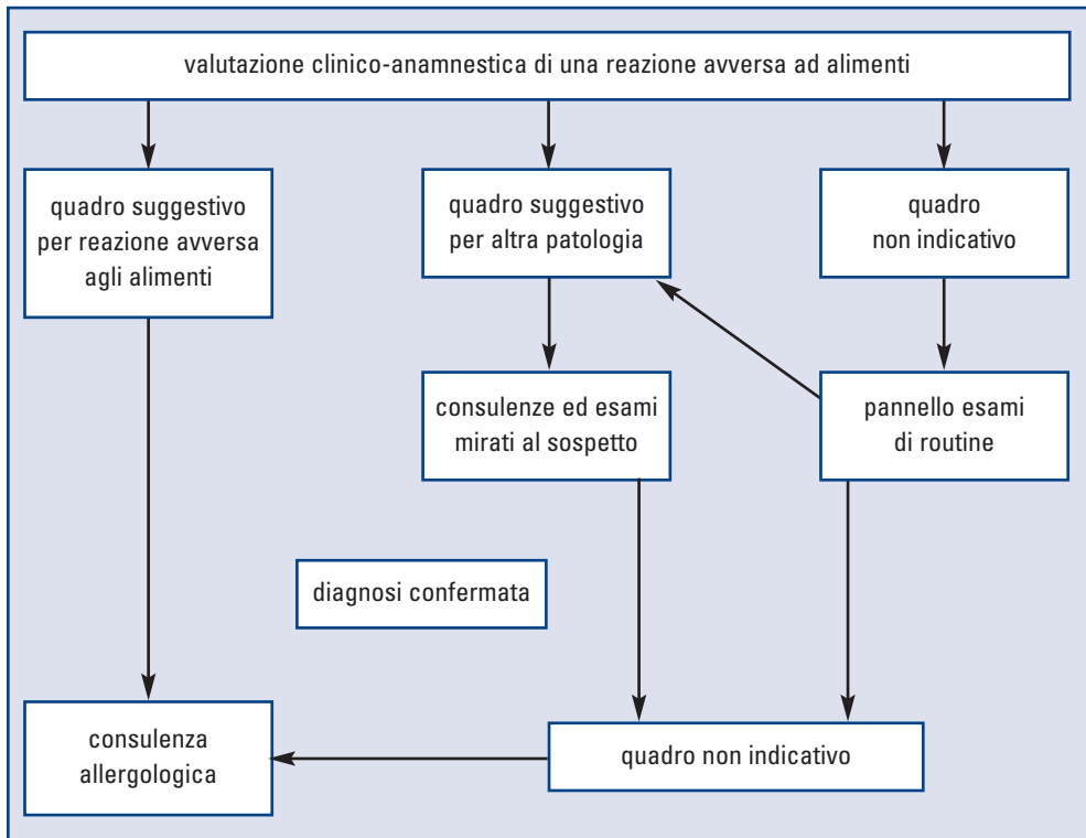
Figura 2. Algoritmo diagnostico.
